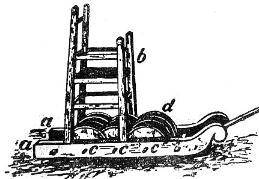
2. ábra. Cséplőszán
